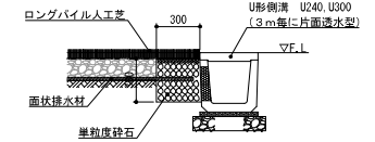
A-A断面図 S=1:20
