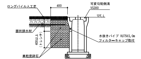
B-B断面図 S=1:20
